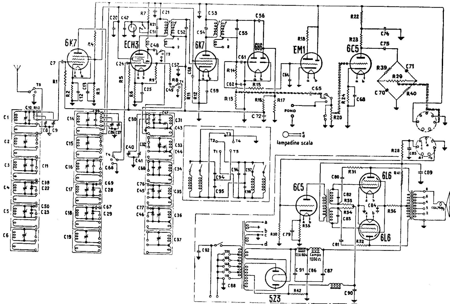
COMPAGNIA GENERALE DI ELETTRICITÀ. — Mod. 919. — Media frequenza: 468 kHz. — (v. Tabella). — 1941-42.
